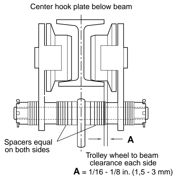
(Dwg. MHP1589)
