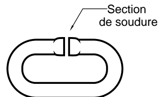
Maillon «C»
