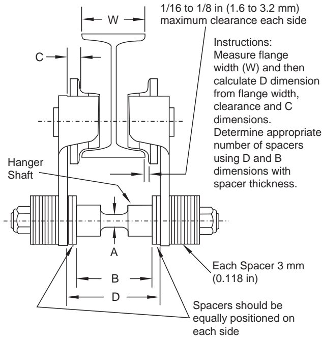
(Dwg. MHP0785)
