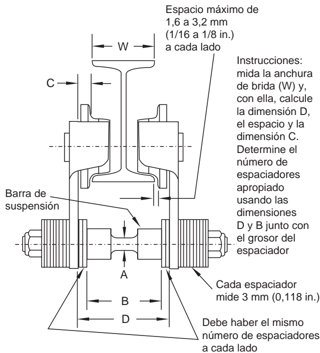
(Dibujo MHP0785E)
