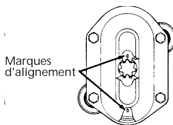
Figure 10 - Alignement d'engrenages
