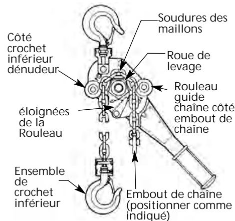
Figure 11 - 3/4, 1, 1 1/2, 2 et 3 tonne
